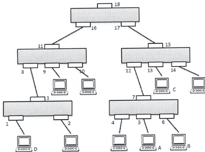
Рисунок 1 – Фрагмент сети
