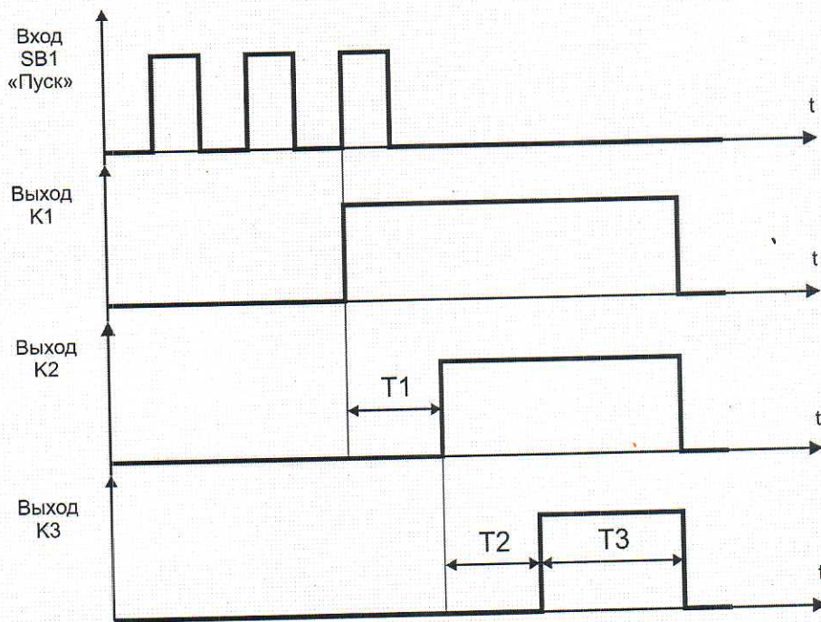
Рисунок 1 – Временная диаграмма
