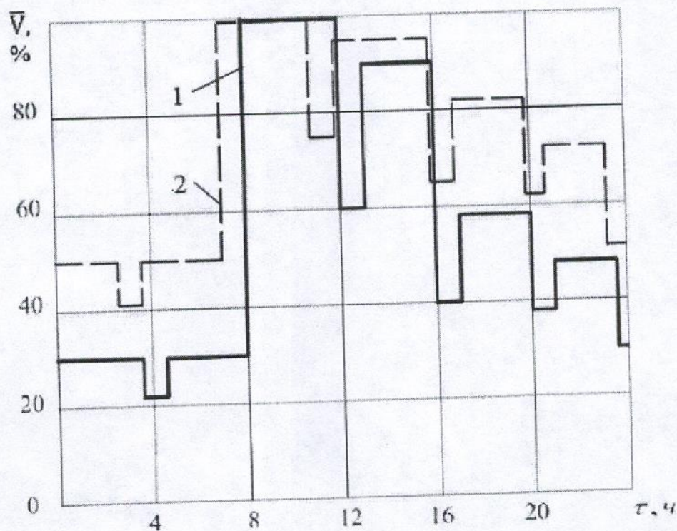
Рисунок 1 – Суточный график безразмерного расхода сжатого воздуха
