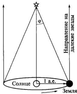
Рис. 2 Схема определения расстояний до далеких звезд методом годичного параллакса
