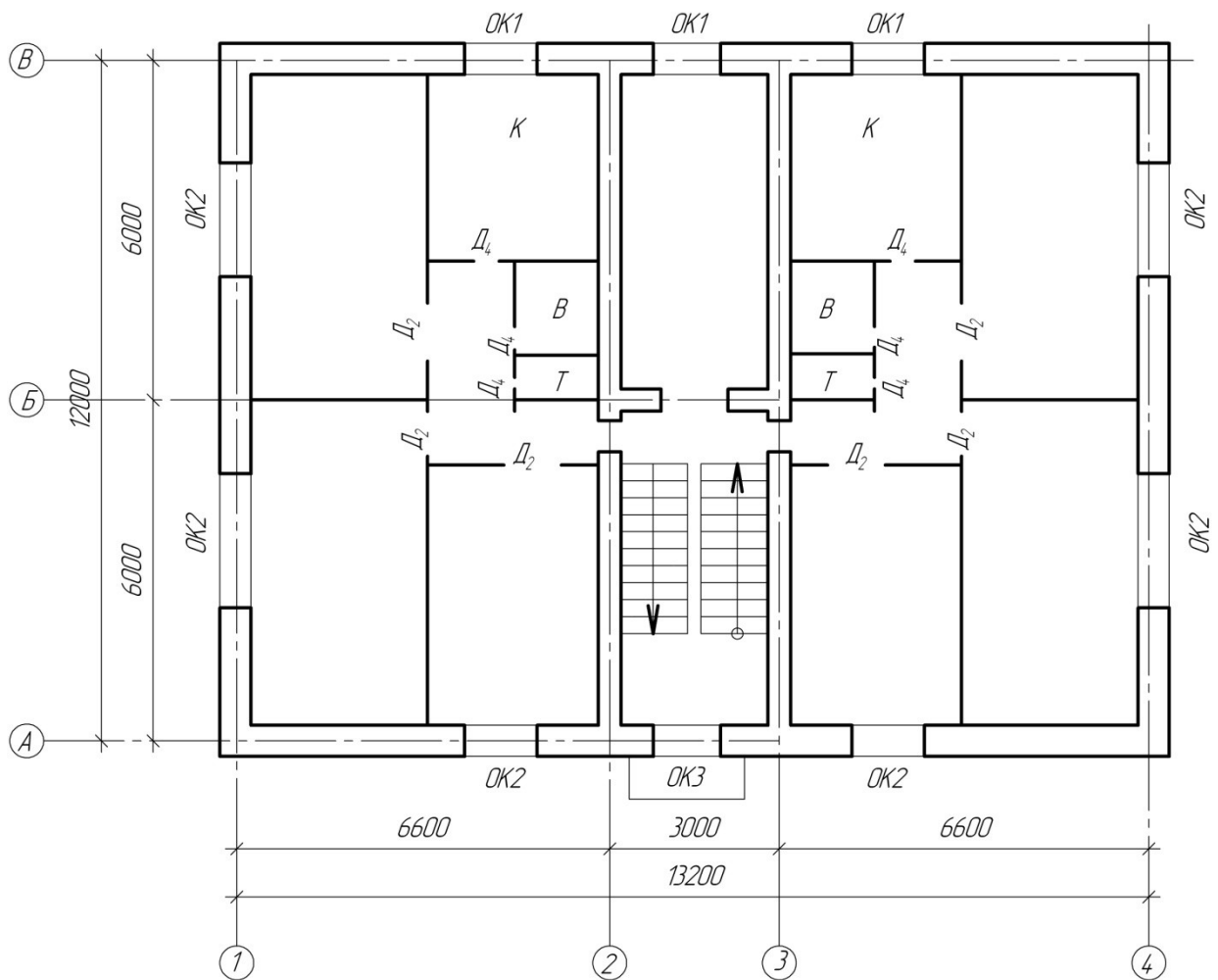
Вариант 7 Схема плана 2 этажа
