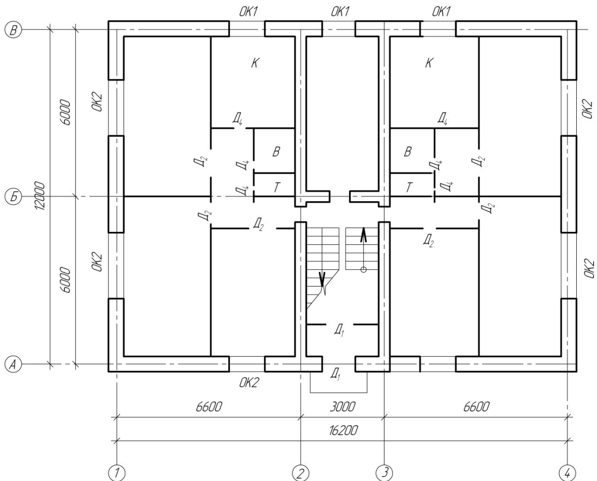
Вариант 6 Схема плана 1 этажа
