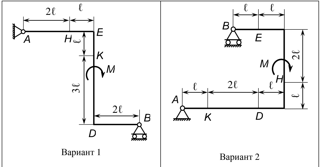
Рисунок 6 – Варианты эскизов жесткой рамы
