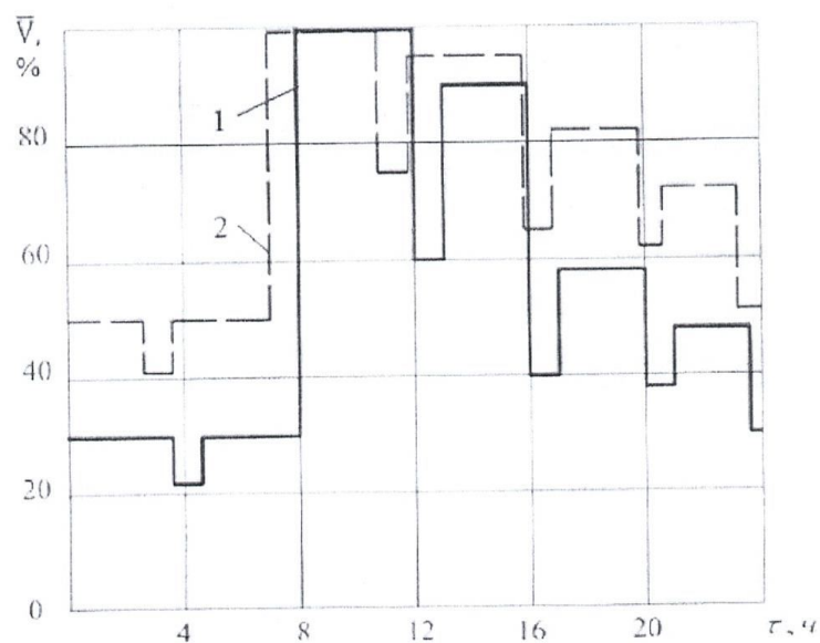
Рисунок 1 – Суточный график безразмерного расхода сжатого воздуха
