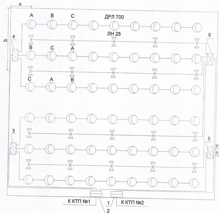
Рисунок – План размещения светильников
