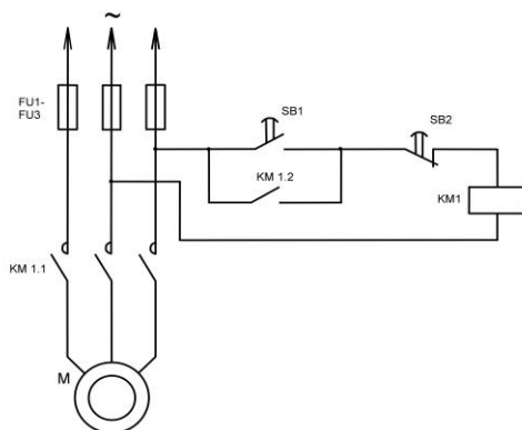
Схема №1
