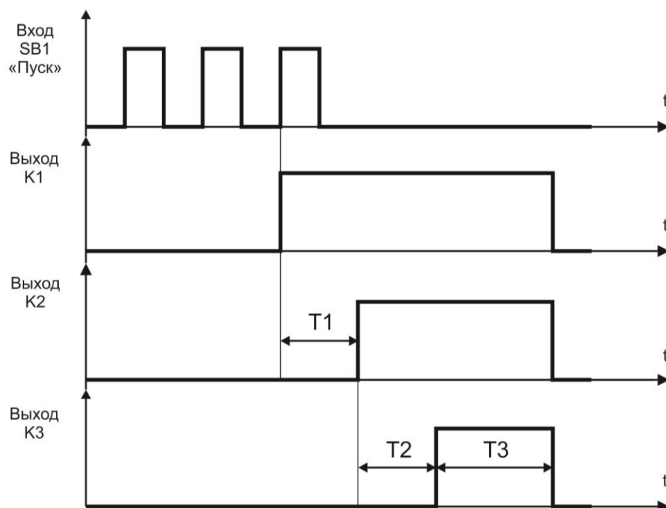
Рисунок 1 – Временная диаграмма
