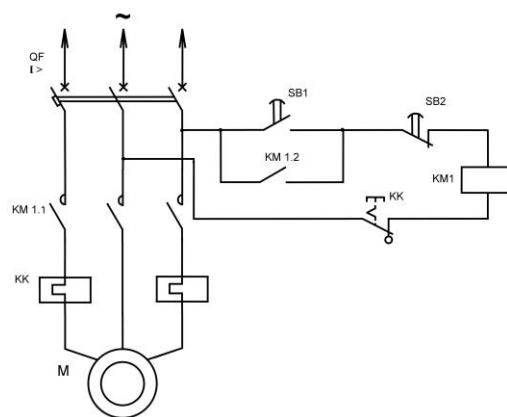
Схема №2
