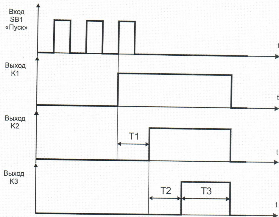
Рисунок 1 – Временная диаграмма
