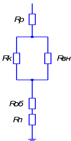
Рисунок 1 – Схема замещения сопротивления человека
