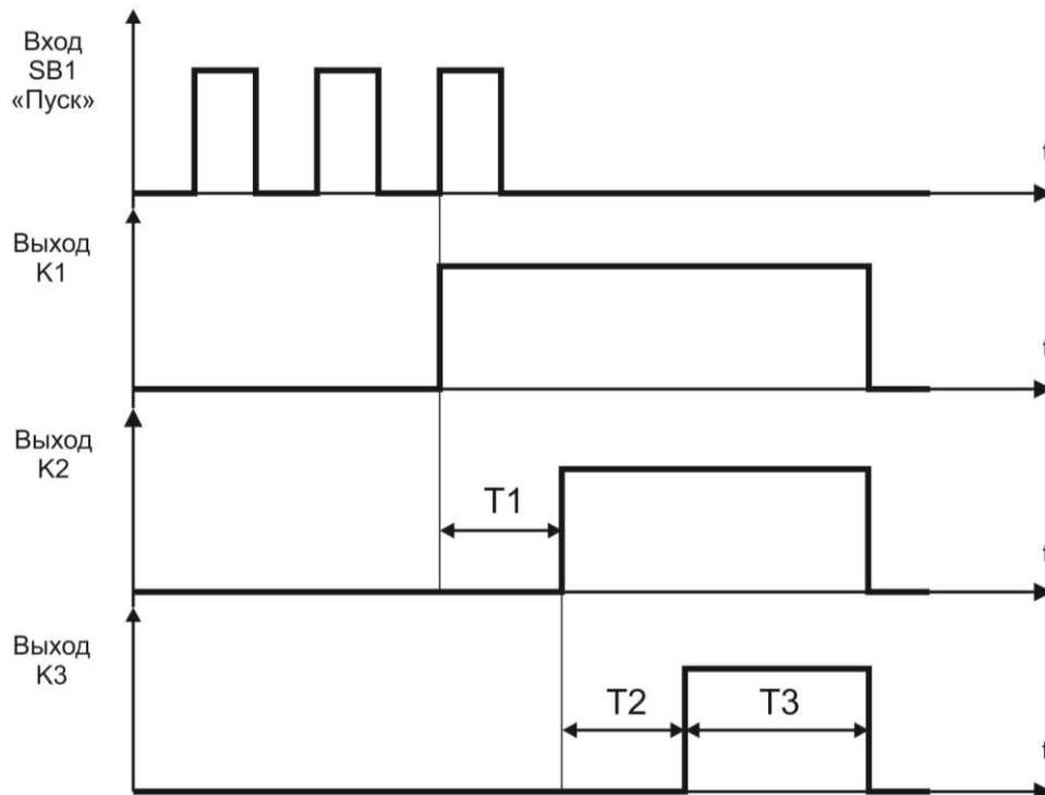
Рисунок 1 – Временная диаграмма
