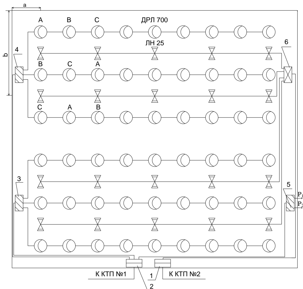
Рисунок – План размещения светильников
