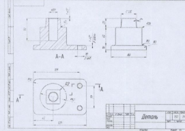
Рис. 1. Чертеж детали
