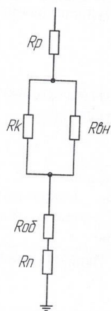
Рисунок 1 – Схема замещения сопротивления человека
