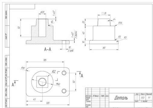
Рис. 1. Чертеж детали
